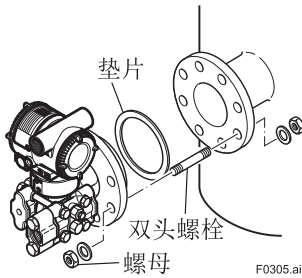
图 3.8 EJ□210□安装
