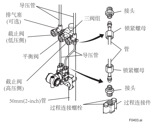
图 4.3 三阀组（配管型）
