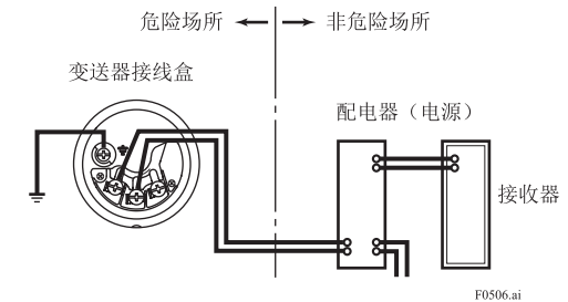
图 5.9 变送器与配电器连接
