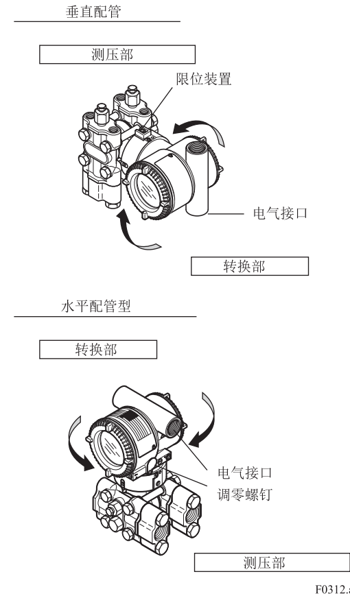
图 3.12 旋转转换部（左侧高压型）
