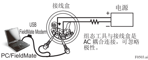
图 5.4 组态工具连接
