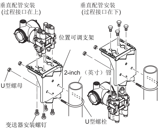
图 3.3 变送器安装（垂直配管）
