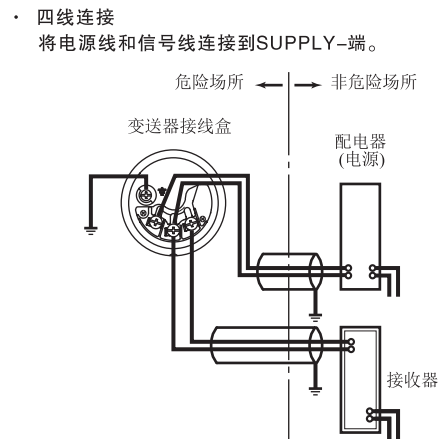
图 5.14 变送器与配电器和接收器连接
