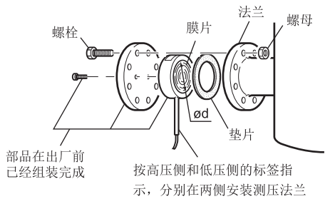
图 3.9 隔膜密封安装
