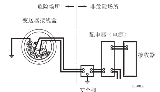
图 5.11 变送器与配电器连接
