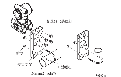
图 3.2 变送器安装（水平配管）
