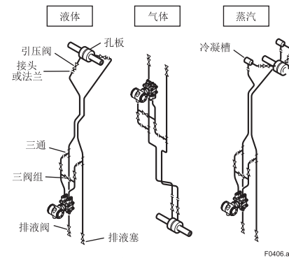
图 4.6 配管示例（差压变送器）
