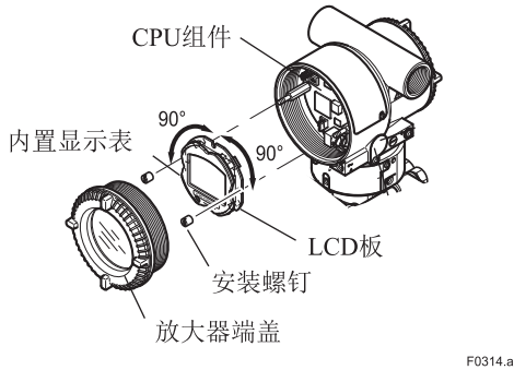
图 3.17 旋转内置显示表
