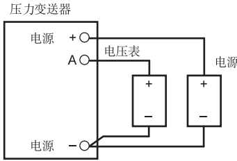
四线连接
