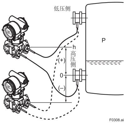
图 3.11 液罐上的安装实例（安装注意）
