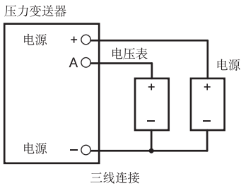
三线连接
