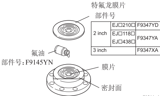
图 3.14 特氟龙膜片粘贴
