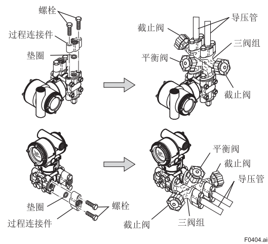
图 4.4 三阀组（直接安装型）
