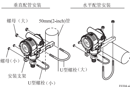
图 3.4 EJ□510□和 EJ□530□安装
