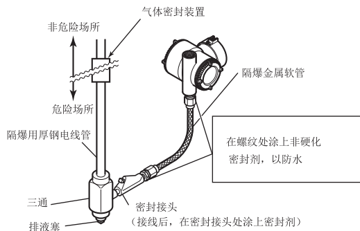
图 5.17 隔爆金属软管典型接线
