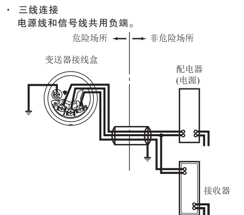
图 5.13 变送器与配电器和接收器连接
