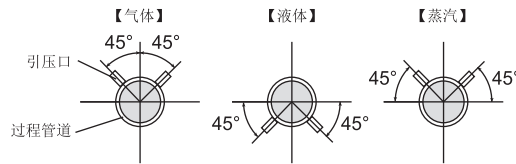
图 4.5 引压口角度（水平安装）
