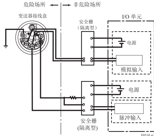
图 5.12 变送器与安全栅和接收器连接
