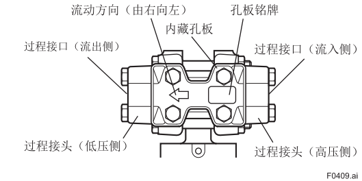
图 4.9 内藏孔板流向示意图
