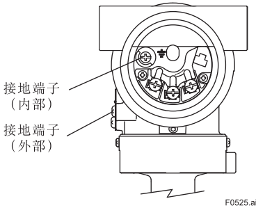
图 5.19 接地端子
