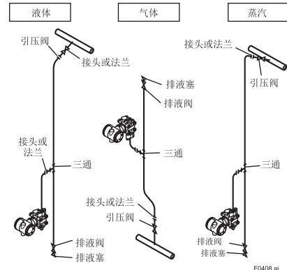
图 4.8 配管示例（表压/绝压变送器）
