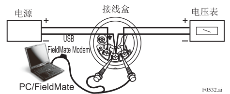
图 5.5 四线连接
