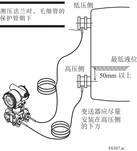
图 3.10 液罐隔膜密封安装
