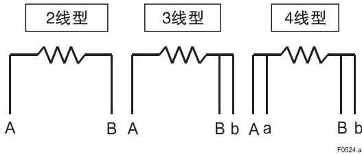
图 5.18 RTD 侧接线方法
