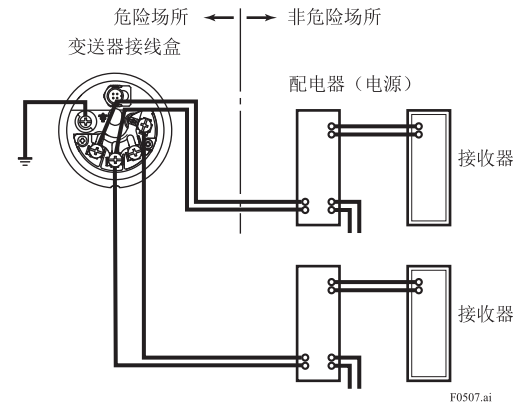
图 5.10 变送器与配电器连接
