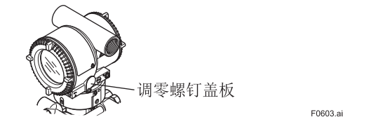
图 6.2 外部调零螺钉
