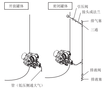
图 4.7 配管示例（EJ□210□）
