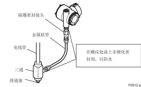
图 5.16 隔爆密封接头典型接线
