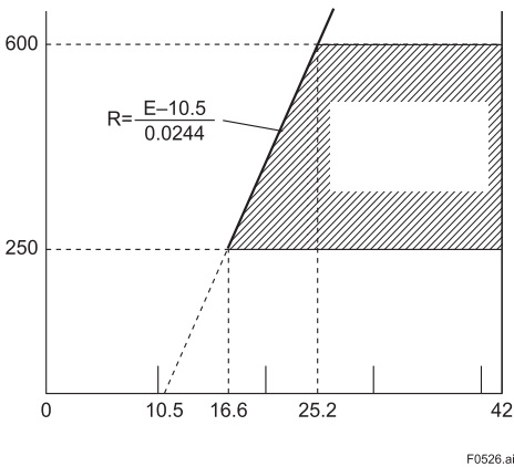
图 5.20 电源电压与外接负载电阻关系图
