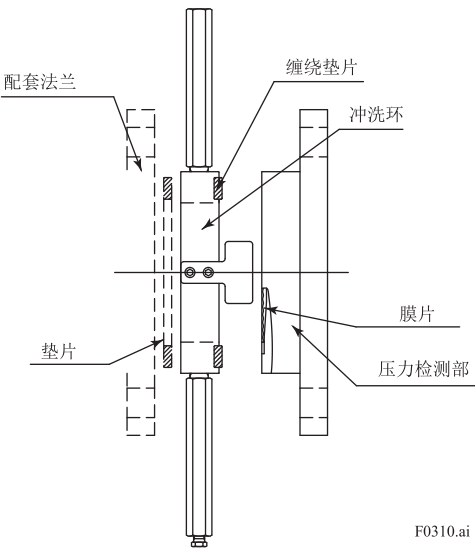
图 3.13 安装到过程法兰
