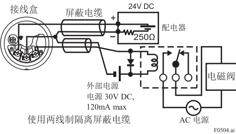
图 5.7 状态输出连接
