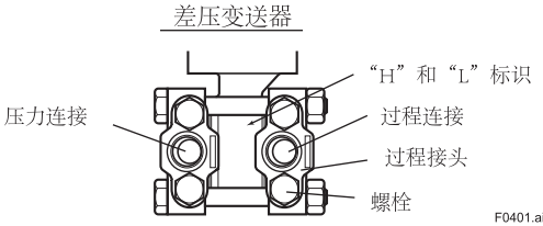
图 4.1 膜盒上的“H”和“L”标记
