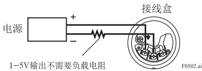
图 5.3 电源连接
