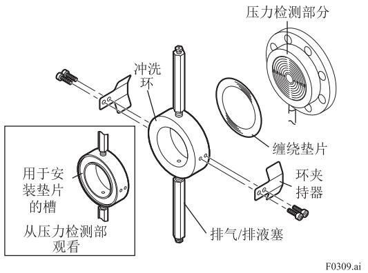
图 3.12 安装到压力检测部
