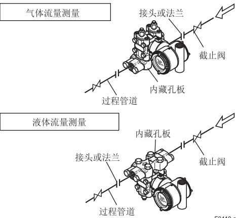
图 4.10 过程管道配管示例 (EJ□115□)
