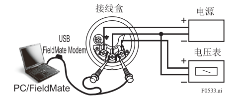
图 5.6 三线连接
