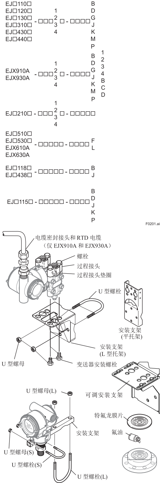
图2.1 变送器安装部件
