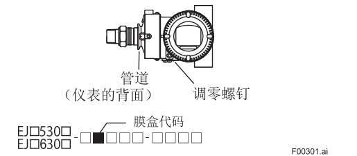
图 3.1 EJ□530□和 EJX630A 水平安装 安装隔膜密封、过程接头或阀组时，请确保在组装之前没有异物附着在垫圈（或O形圈）的密封面上。如有异物附着，可能会导致泄漏。
